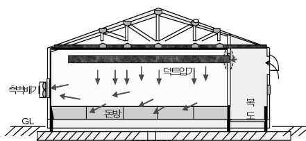
(측벽 덕트 입기 → 측벽 배기)
