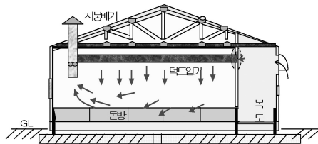
(측벽 덕트 입기 → 지붕 배기)
