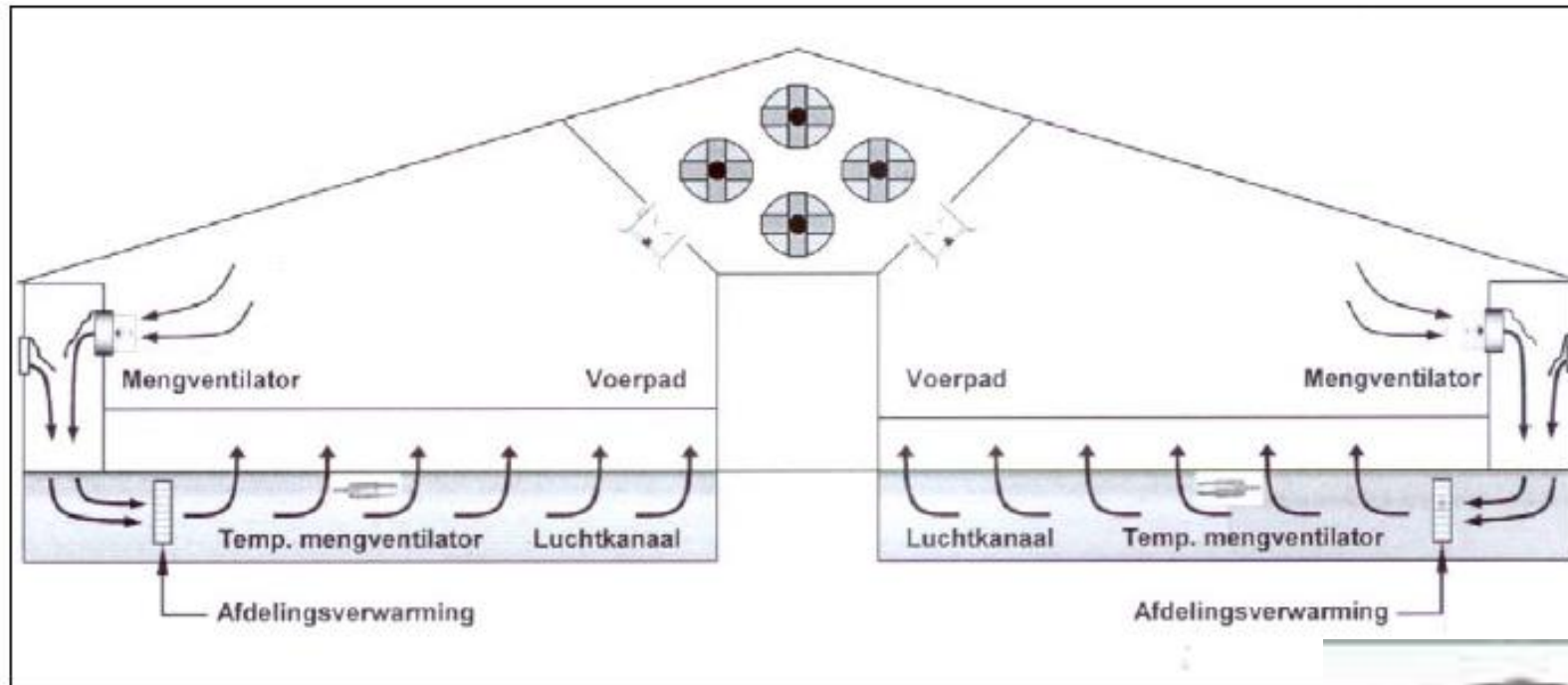
Figuur 43 Mengventilatie
